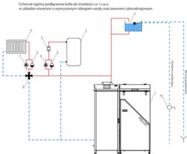
1. Kocioł Ball Eco 2. Naczynie wyrównawcze z zaworem 3. Zawórki CWU 4. Odbiornik ciepła w obrotu CO 5. Zawór Czterodrogowy 6. Zawór obrotowy CO 7. Pompa obrotowa CO 8. Pompa obrotowa CWU 9. Zawór Czterodrogowy
